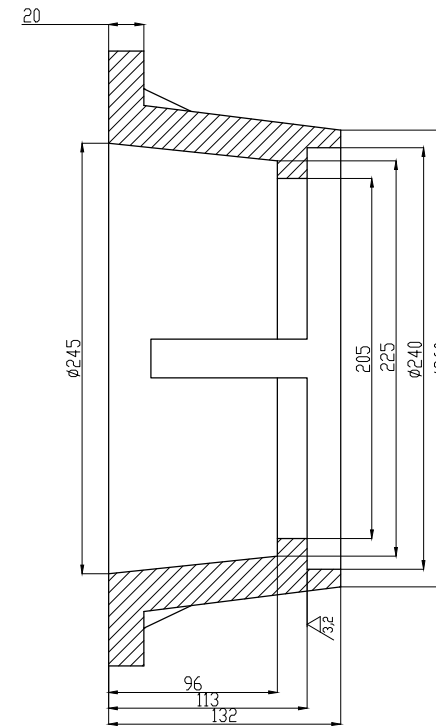
SECÃO B-B ESCALA 1 : 1.5
