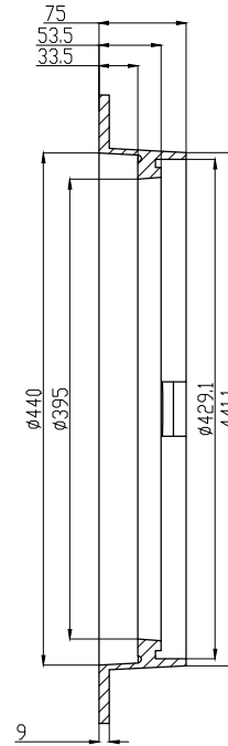
SECÃO A-A ESCALA 1 : 2.5
