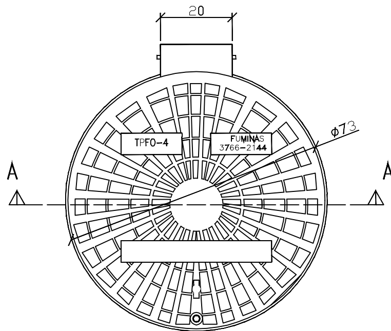
VISTA SUPERIOR DA TAMPA
