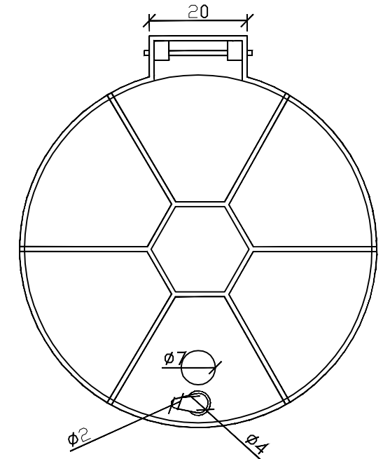
VISTA INFERIOR DA TAMPA
