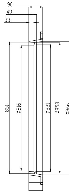
SEÇÃO A-A ESCALA 1 : 5
