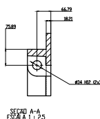
SEÇÃO A-A ESCALA 1:1,25
