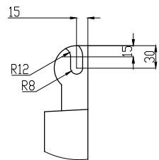
DETALHE A ESCALA 2 : 5
