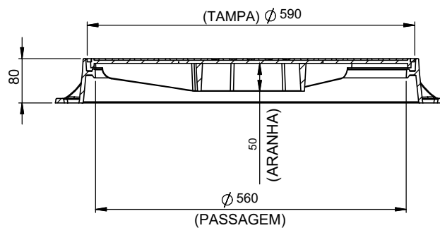
SEÇÃO A-A ESCALA 1 : 6
