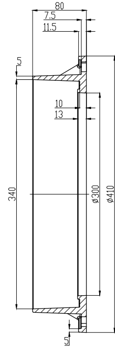
SECÃO A-A ESCALA 1 : 2
