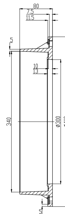
SECÃO A-A ESCALA 1 : 2
